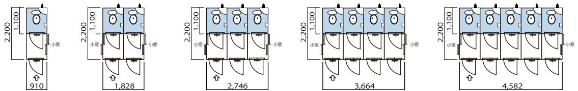
KT-1型 KT-2型 KT-3型 KT-4型 KT-5型
