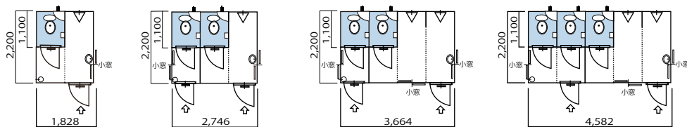
KT-9型 KT-10型 KT-11型 KT-12型
