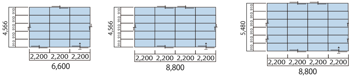
KJW-15連棟 KJW-20連棟 KJW-25連棟
