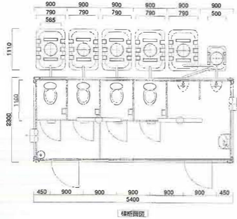
RQMS-8型 シャトレ水洗式 寸法 W5,400 x D2,300 x H2,595
