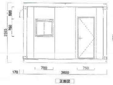
RQ-2型 水洗式 寸法 W3,600 x D2,300 x H2,595
