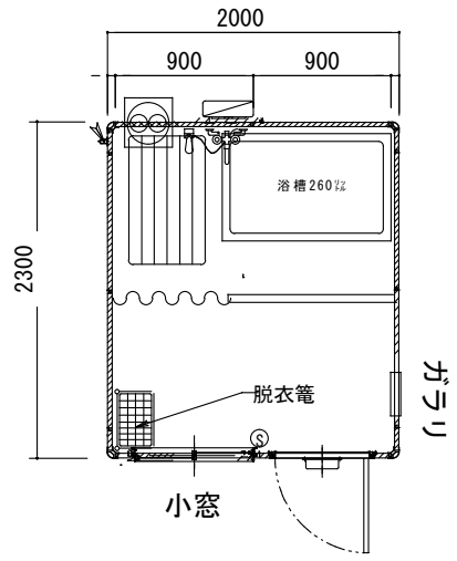
平面図
