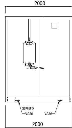
背面図
