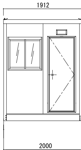
正面図
